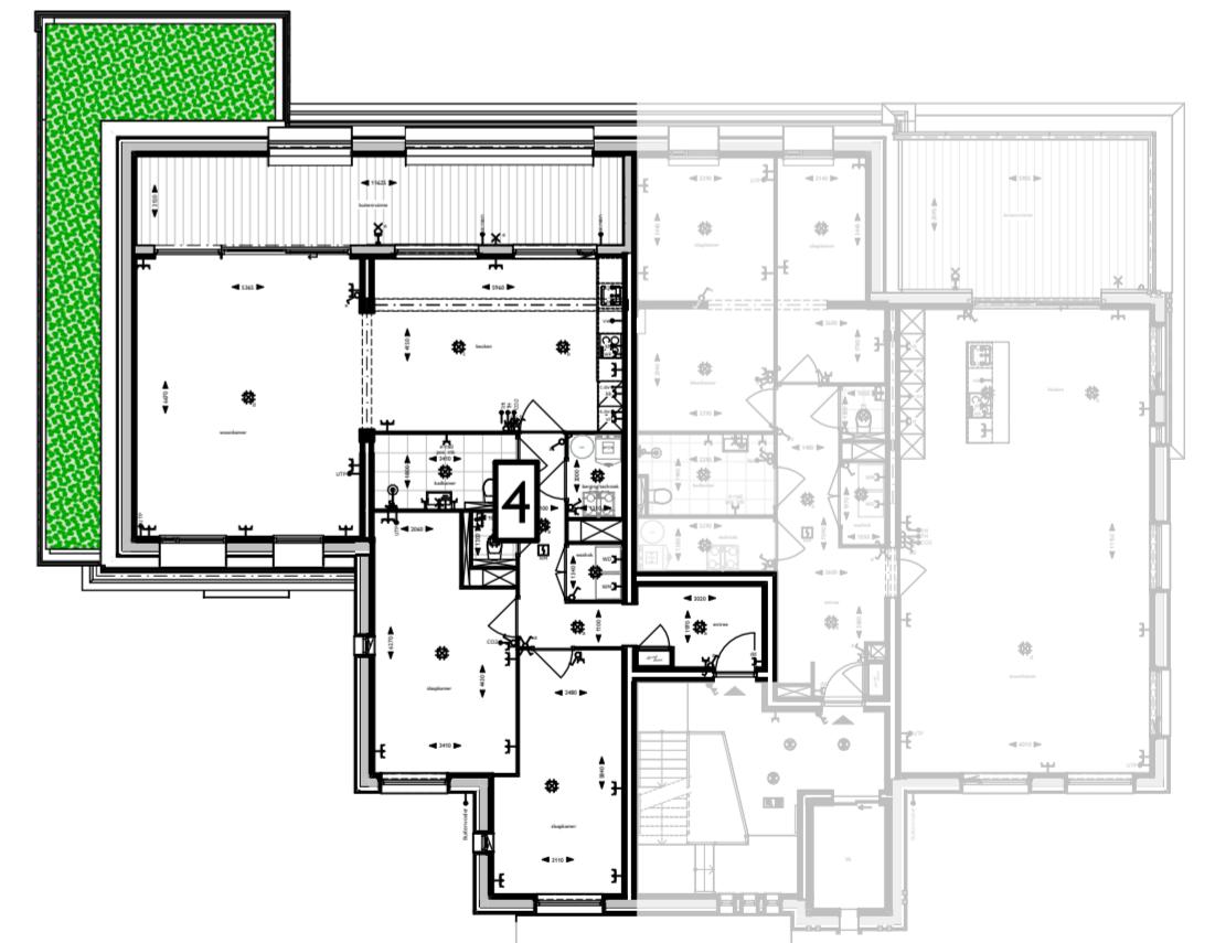
1e verdieping
